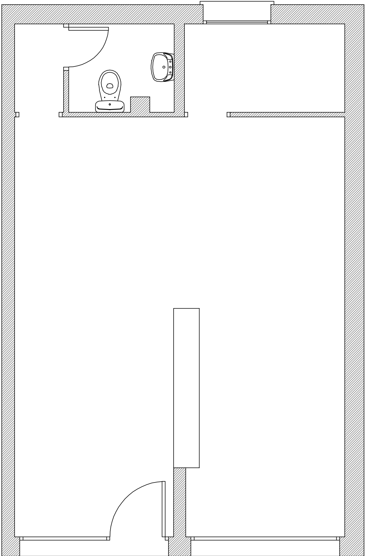
Planta Baixa
